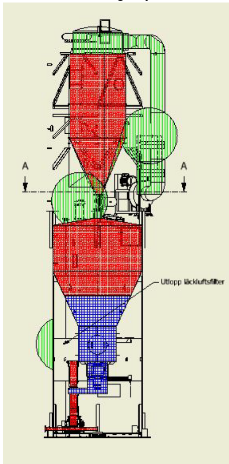
Zonindelning; Träpulversilo
