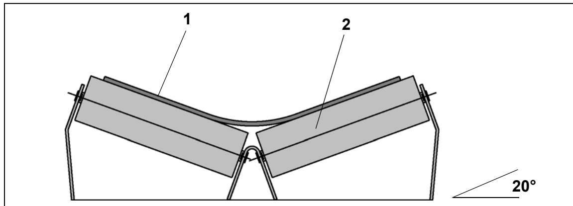
Transportbånd og bærerullestasjon ved båndbredde 500
